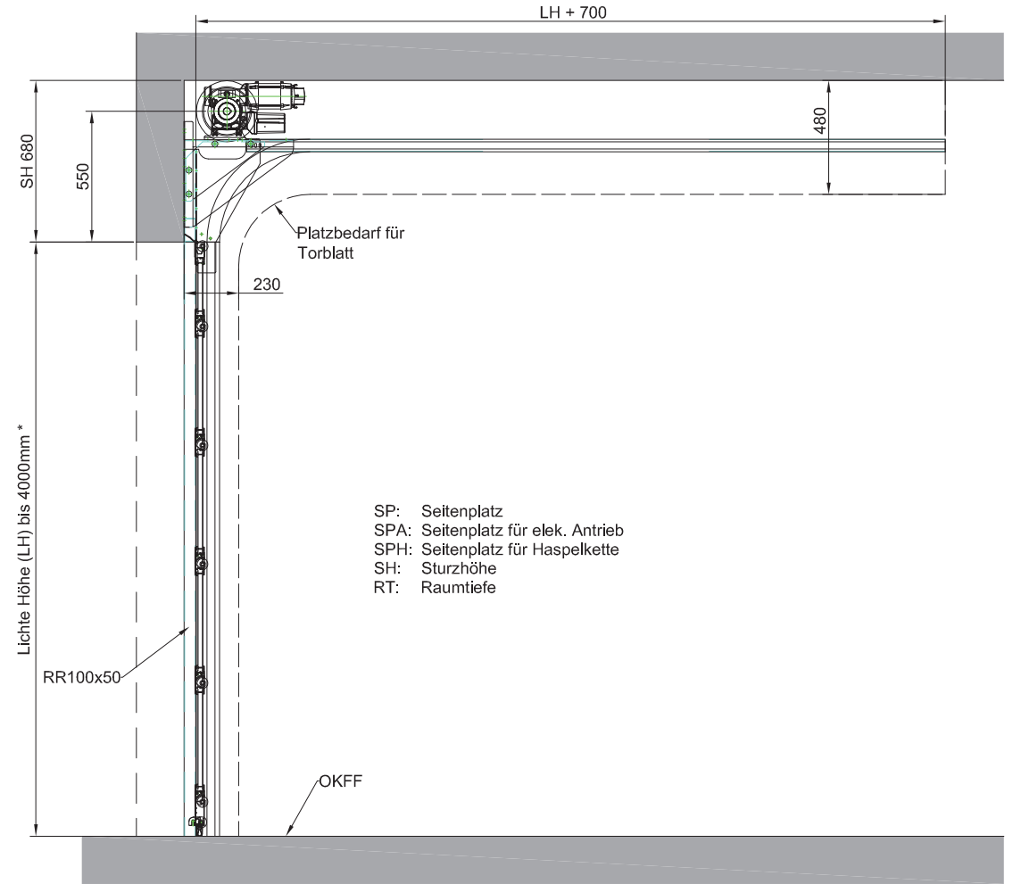
Vertikalschnitt
