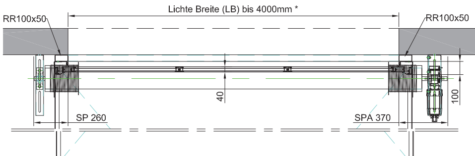
Horizontalschnitt
